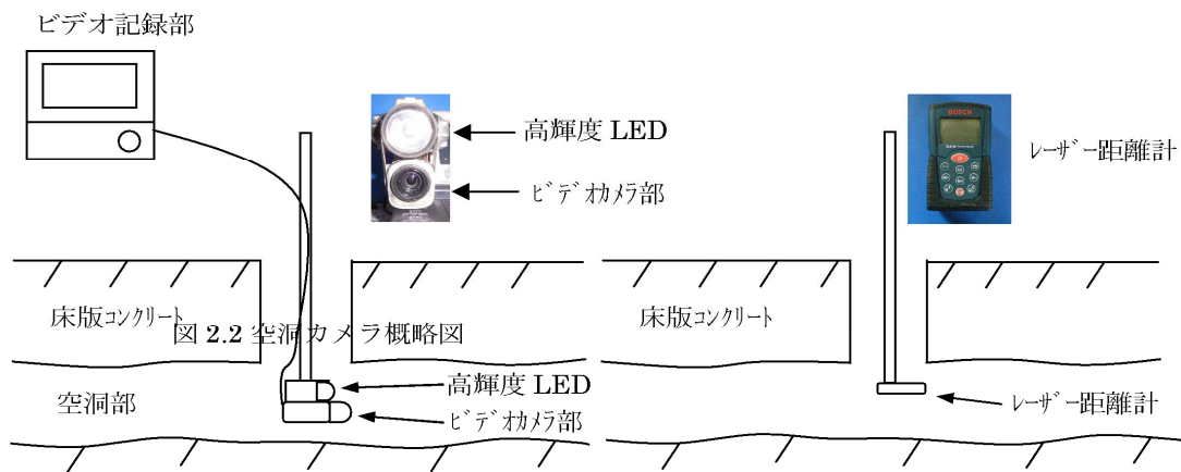
③床底の空洞内測距
