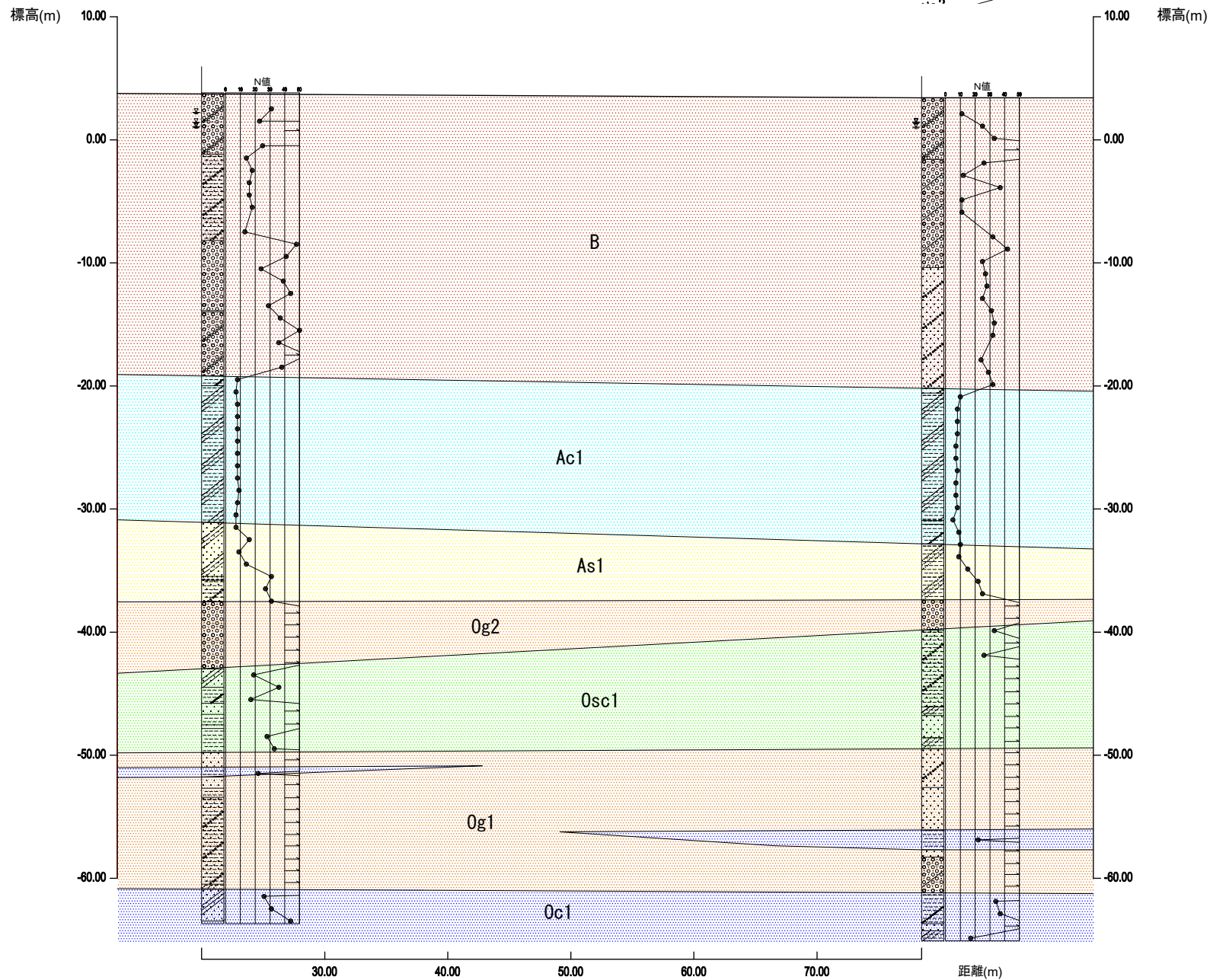
地盤調査で判明した地層断面図
