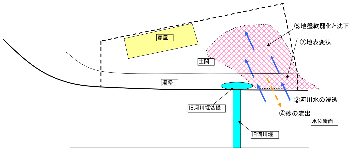
旧河川堰と変状の平面図
