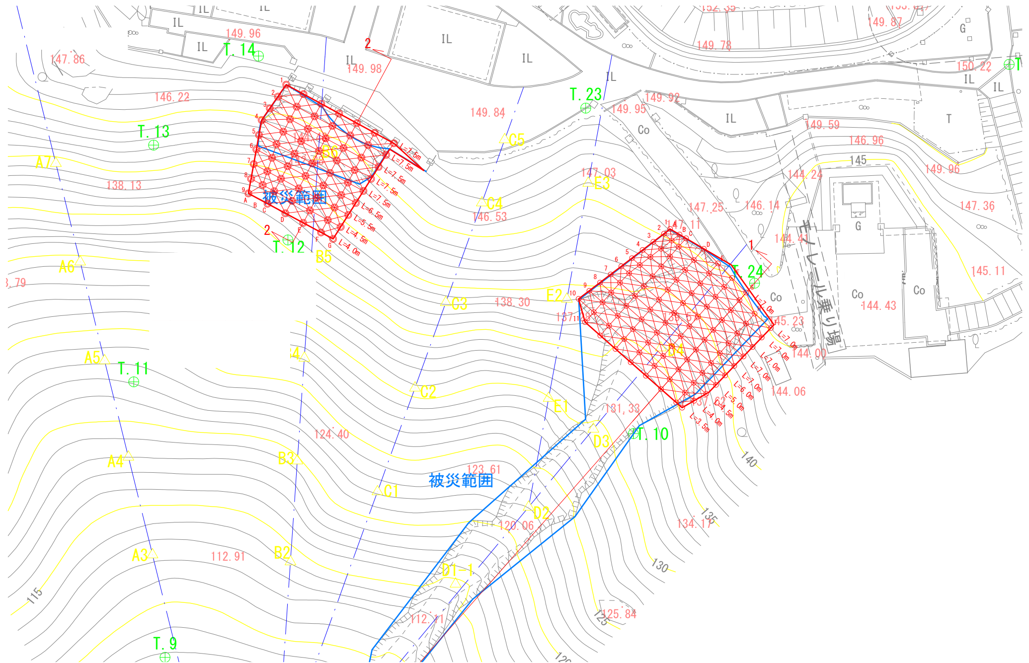
斜面復旧対策工の計画事例
